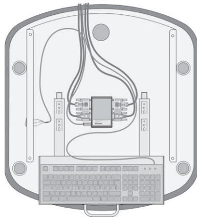
Switch Box GM3 auf Zwischenboden montiert.
