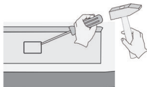
Montageöffnung Monitorschalter freilegen
